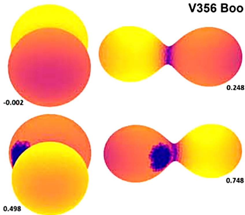
Structure géométrique de V356 Boo obtenue à partir de l'étude des courbes de lumière et à l'aide du logiciel PHOEBE - d'après Poro et al. 2022
