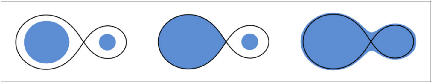
Les différents types de binaires à éclipses : EA détachées - EB semi-détachées - EW en contact Les lignes noires représentent les lobes de Roche
