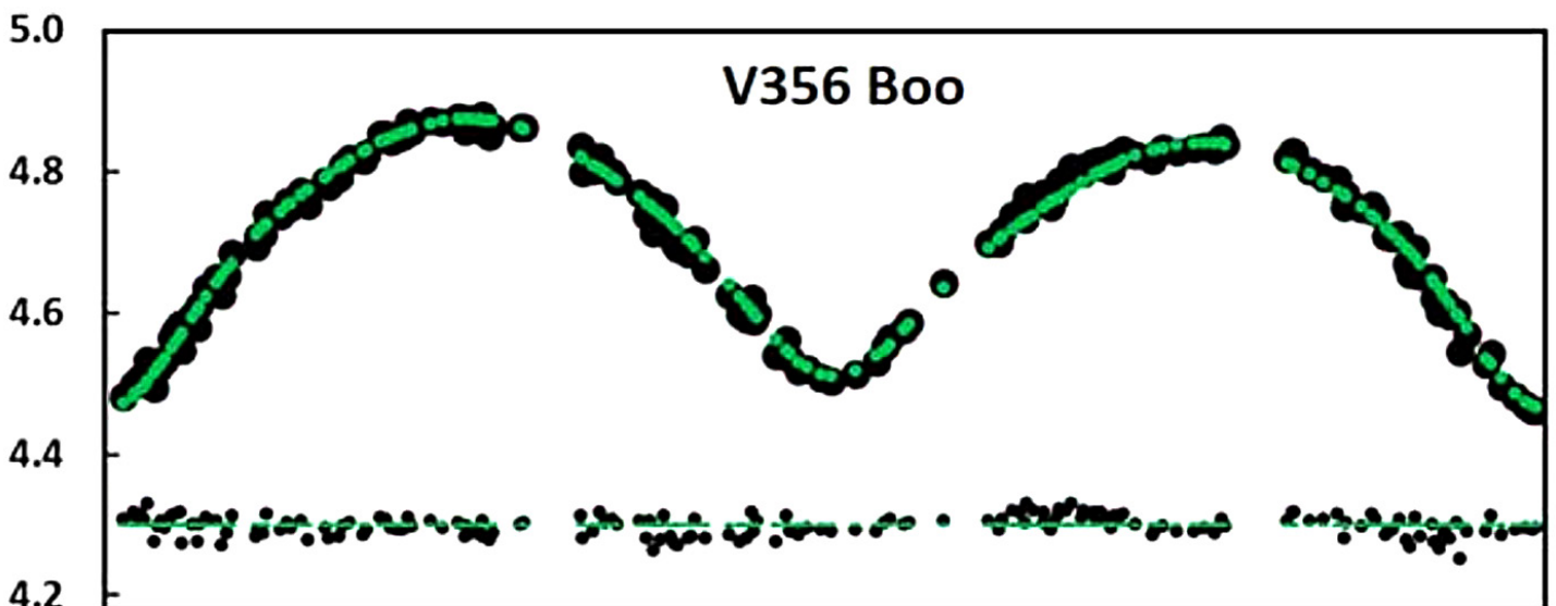
Courbe de lumière de V356 Boo en bande V d'après Poro et al. 2022
